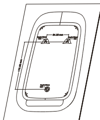
Modello di installazione X1
