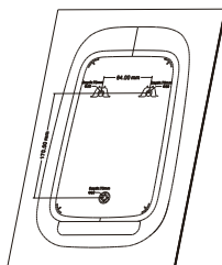
Modèle d'installation X1
