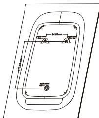
Modelo de instalação X1
