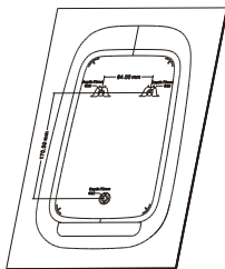
Installatiesjabloon X1
